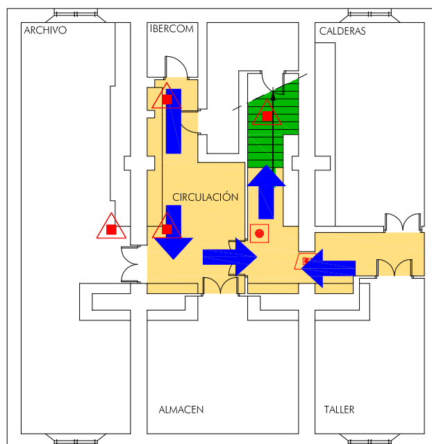
PLANTA SÓTANO
