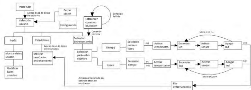
Figura 1. Diagrama de bloques del sistema.
