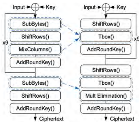
Figura 1. Representación esquemática de AES: a) Estándar, b) Basado en T-box.
