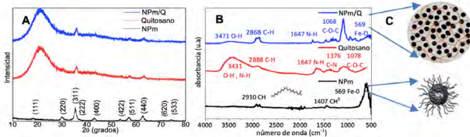
Figura 1: A) Diagramas de DRX de las NPM del quitosano y de las nano-cápsulas de NPM/Q. B) Espectros FTIR de las NPM, del quitosano y de las NPM/Q. C) Diagrama de las NPM/Q (superior) y de las NPM (inferior)
