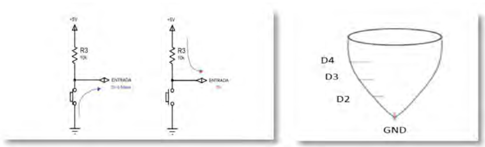
Figura 2. Sensor de nivel de llenado.
