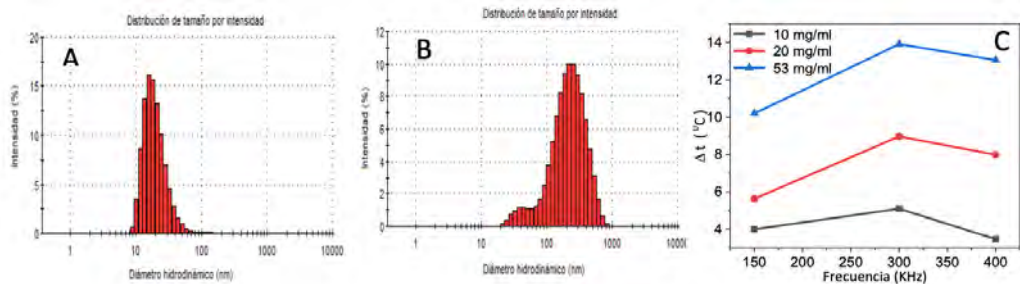
Figura 2. Distribución de tamaño de partículas mediante dispersión dinámica de la luz, (A) NPM, (B) NPM/Q, (C) Estudio de hipertermia magnética de las NPM.
