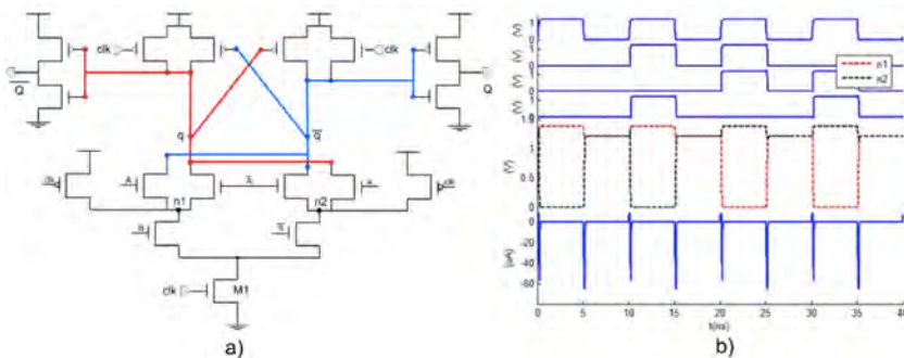
Figura 3. Estructura propuesta y simulación eléctrica de los nodos internos.
